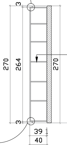
חתך א-א
