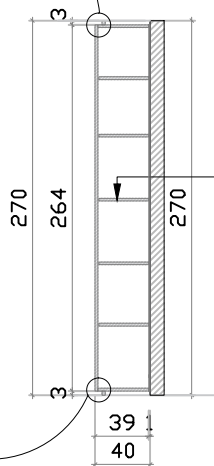
חתך א-א
