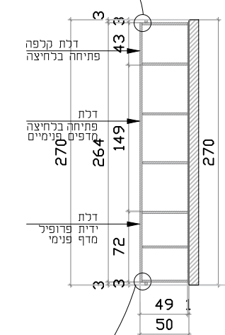
חתך א-א
